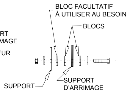
SÉQUENCE DE BOULONNAGE CÔTÉ PASSAGER FIGURE 3
