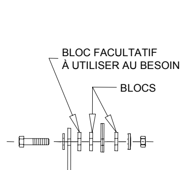
SÉQUENCE DE BOULONNAGE CÔTÉ CONDUCTEUR FIGURE 2
