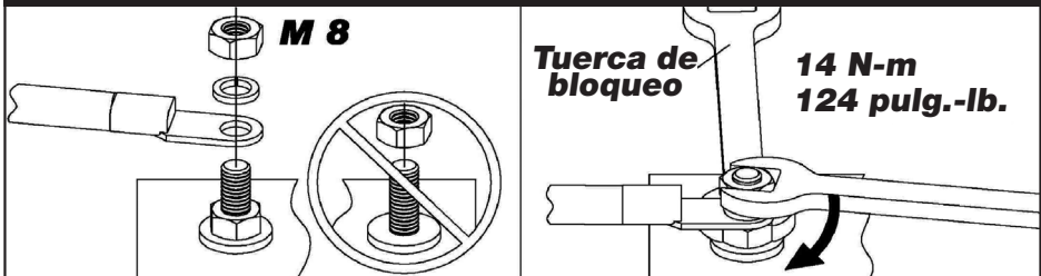
Figura 2: Especificación de torsión
