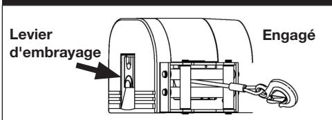
Figure 6 - Engager l'embrayage
