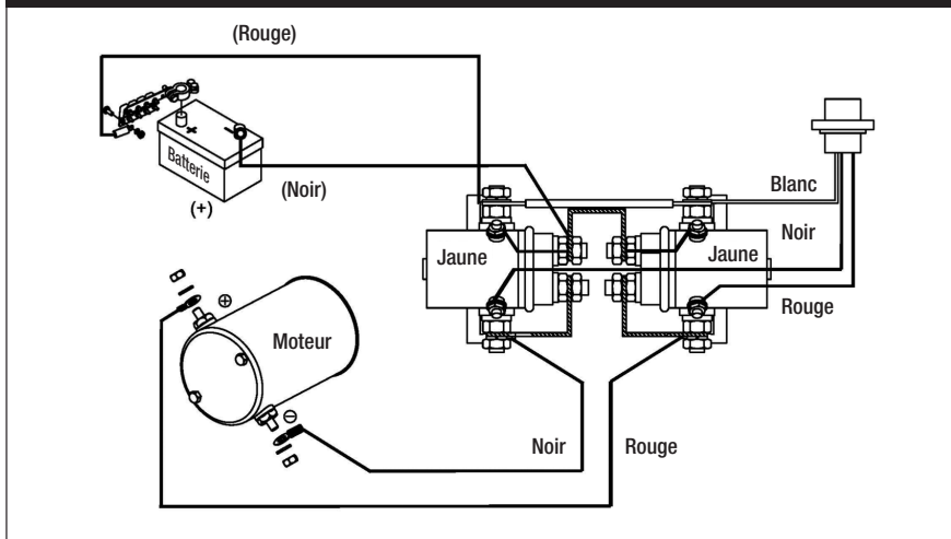
Figure 3 - Schéma de câblage - DC2500, DC3500 et DC4500
