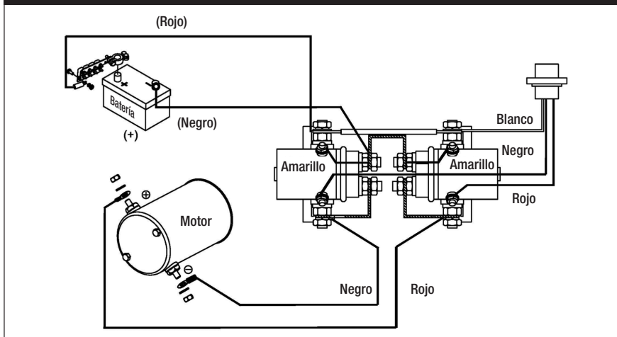
Figura 3: Diagrama del cableado del DC2500, DC3500 y DC4500
