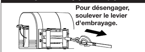
Figure 7 - Désengager l'embrayage
