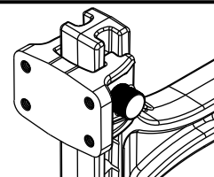
Montage pour crochet d'attelage N/P : 63072
