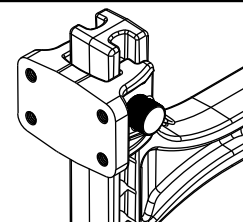
Montaje de pivote P/N: 63072
